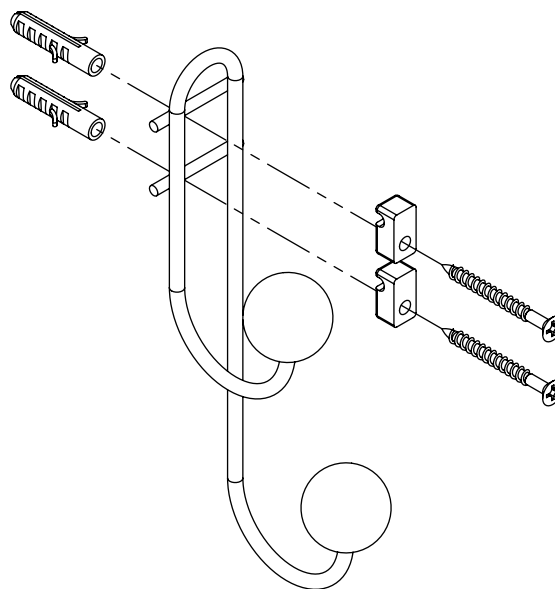
Opção 2 Fixação em parede
