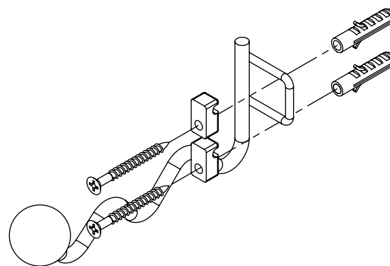
Opção 2 Fixação em parede
